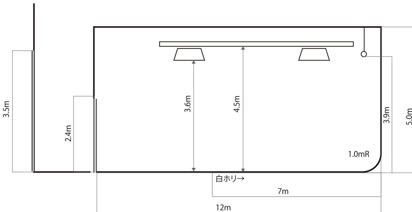
↓立面図
