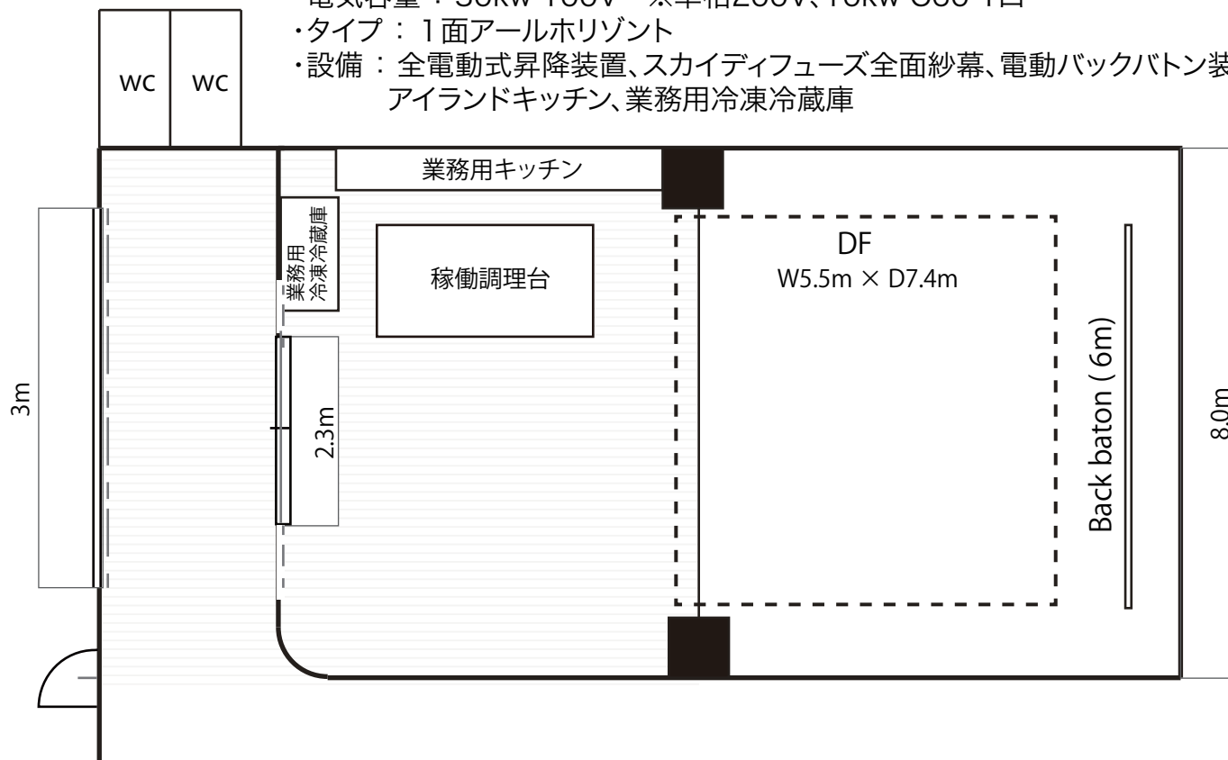
↑俯瞰図
